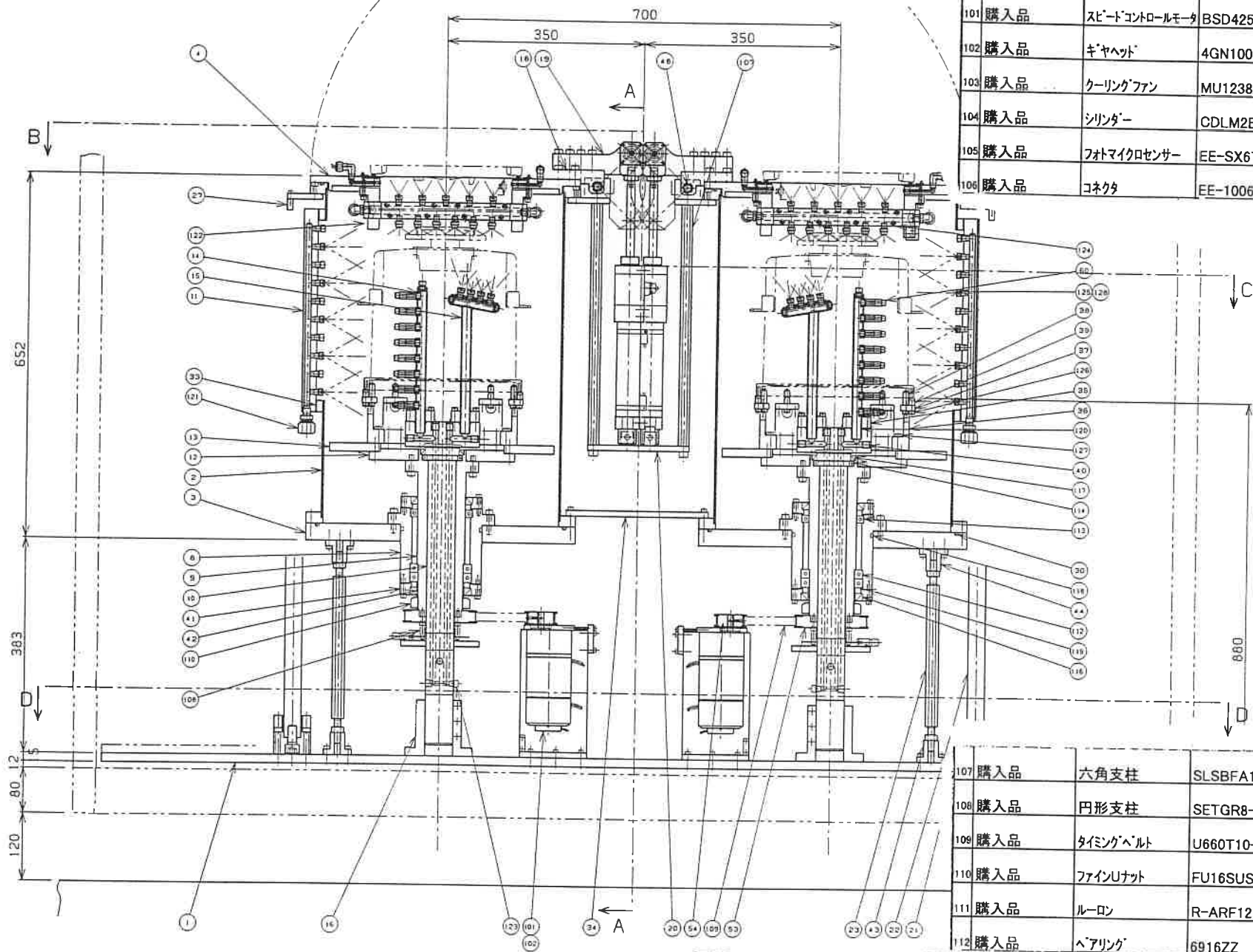
正面断面図
